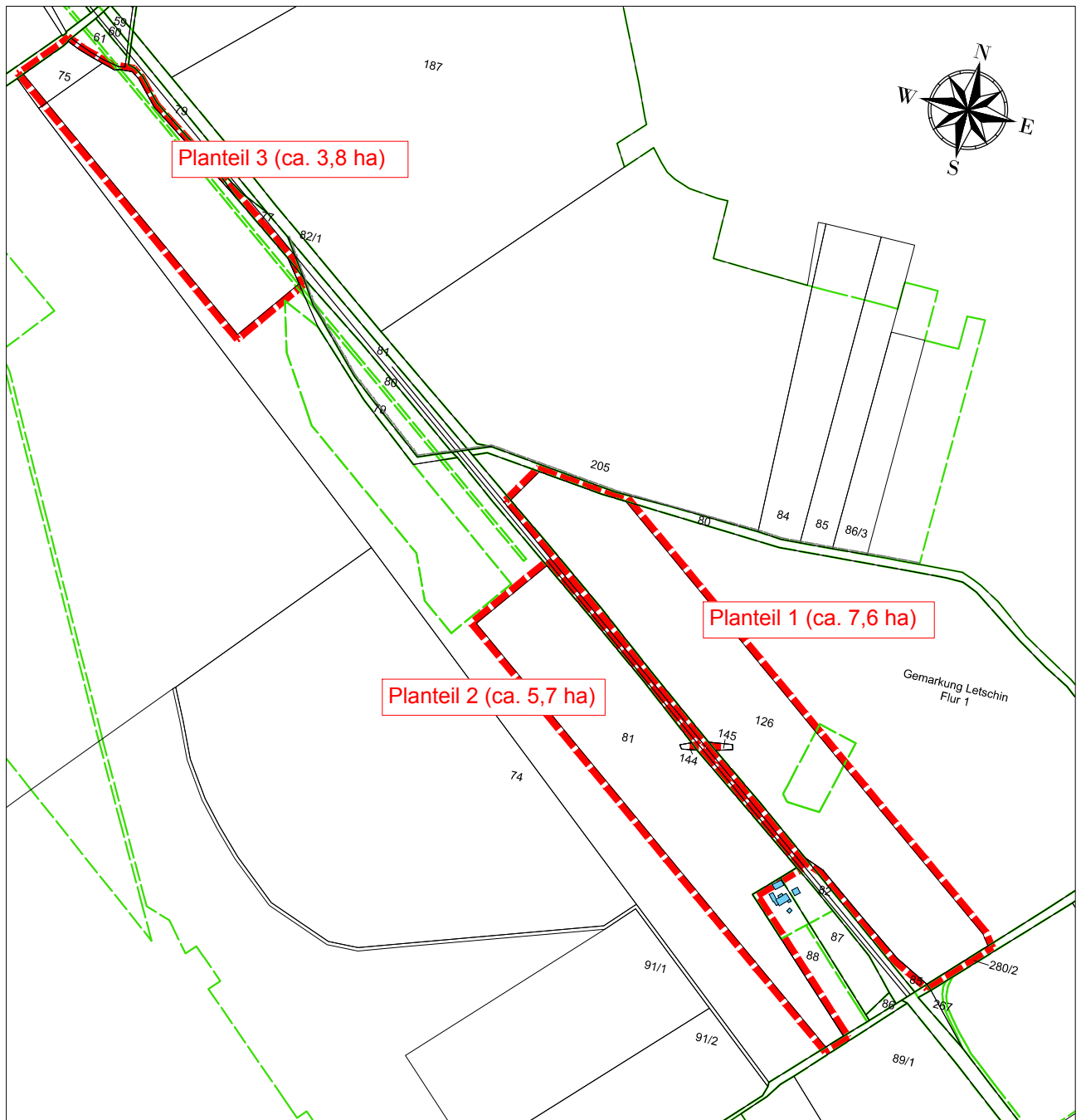
Bebauungsplan Nr. 10 der Gemeinde Letschin "Solarpark Letschin" - Ausgrenzung -
